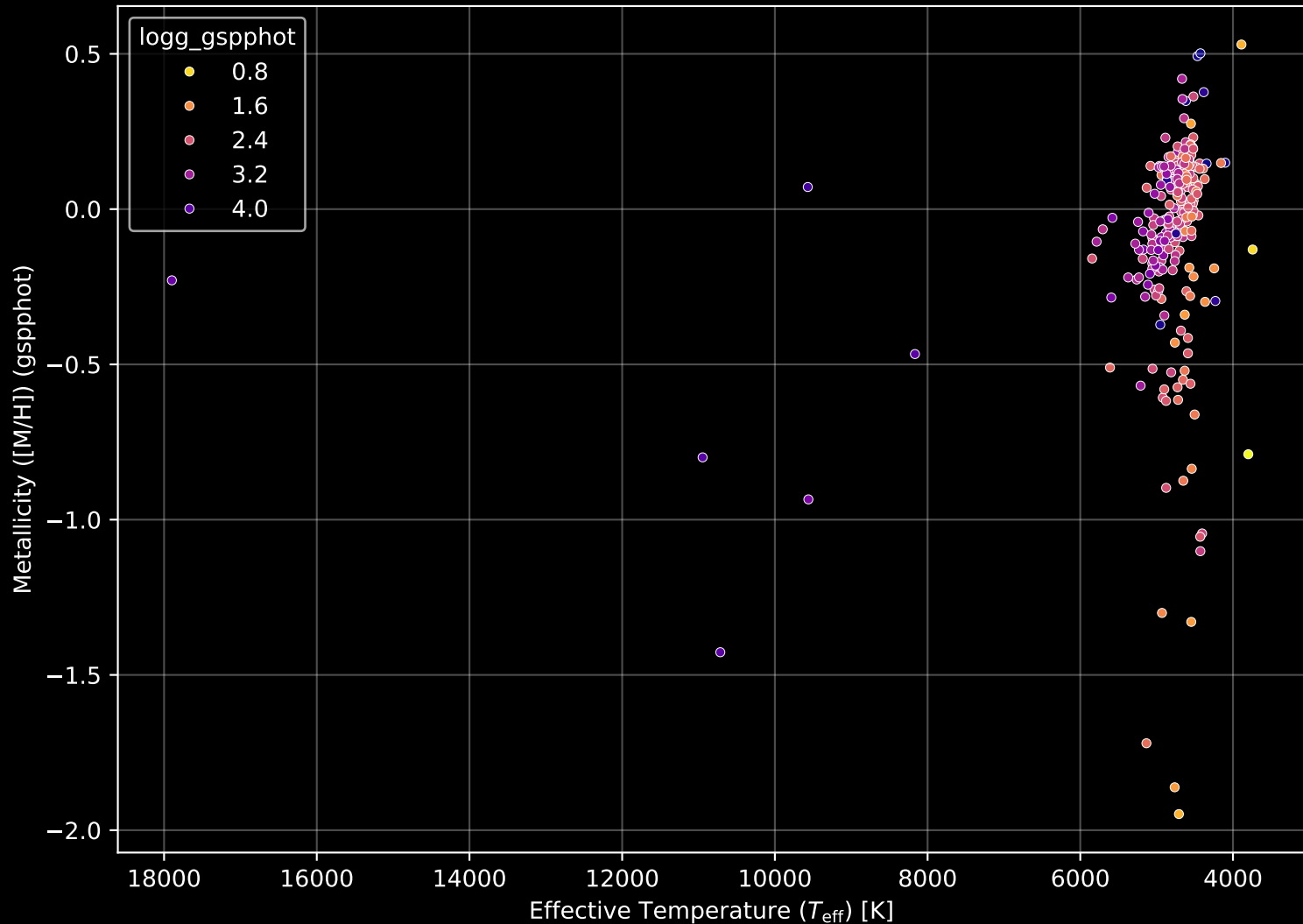
APOGEE DR17 Field: [079-06] Stellar Population Parameters (n= 246)
